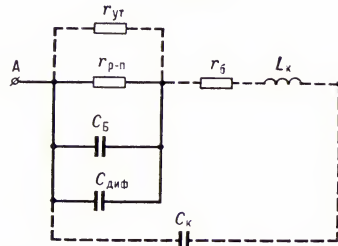
Рис. 3. Малосигнальная (для низких уровней сигнала) эквивалентная схема полупроводникового диода с p-n -переходом: r_{p-n} — нелинейное сопротивление p-n -перехода; r_б — сопротивление объёма полупроводника (базы диода); r_с — сопротивление поверхностных утечек; C_б — барьерная ёмкость p-n -перехода; C_{диф} — диффузионная ёмкость, обусловленная накоплением подвижных зарядов в базе при прямом напряжении; C_к — ёмкость корпуса; L_к — индуктивность токоподводов; А и Б — выводы. Сплошной линией показано подключение элементов, относящихся к собственно p-n -переходу.
